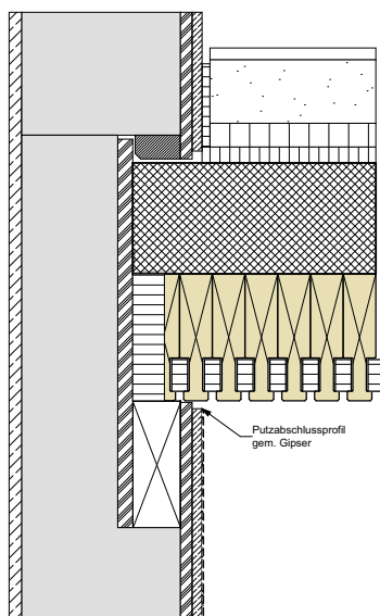
Wandaufleger längs
