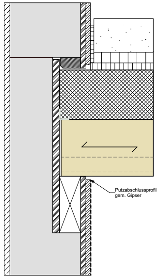
Auflager Aussenwand
