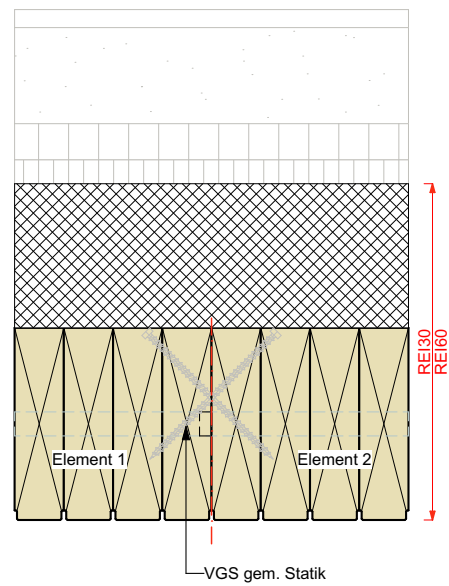
STRATTURA AUTHENTIK Holz-Beton-Verbund
