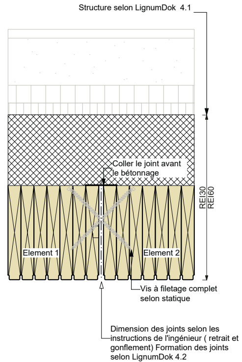
STRATTURA ECO / SHERPA Structure mixte bois-béton
