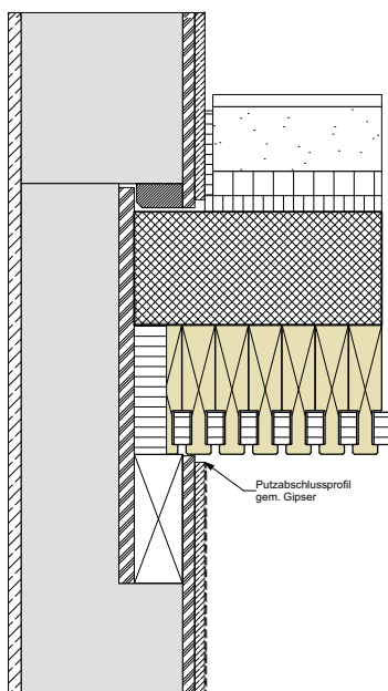
Wandaufleger längs
