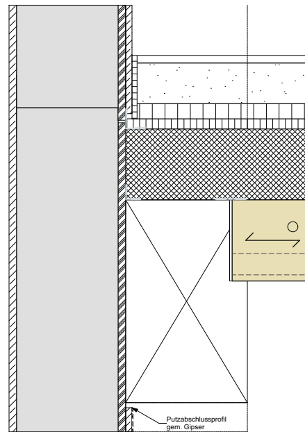
Auflager Träger/Unterzug
