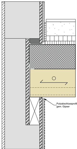
Auflager Aussenwand
