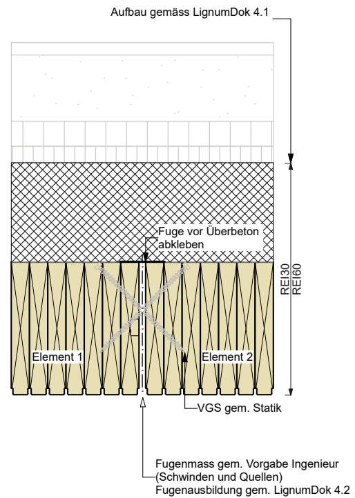
STRATTURA ECO / SHERPA Holz-Beton-Verbund
